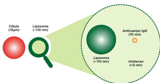
Figura 1. Esquema a escala de irinotecan
